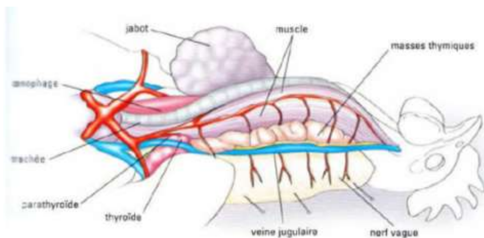
Figure 02: Poulet, vue latérale gauche des organes cervicaux en place (Guérin et al., 2011).
