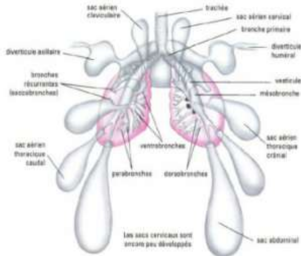
Figure 05: Les sacs aériens de poule (Guérin et al., 2011).
