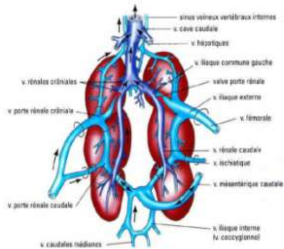
Figure 07: Le système porte rénal (Guérin et al., 2011).
