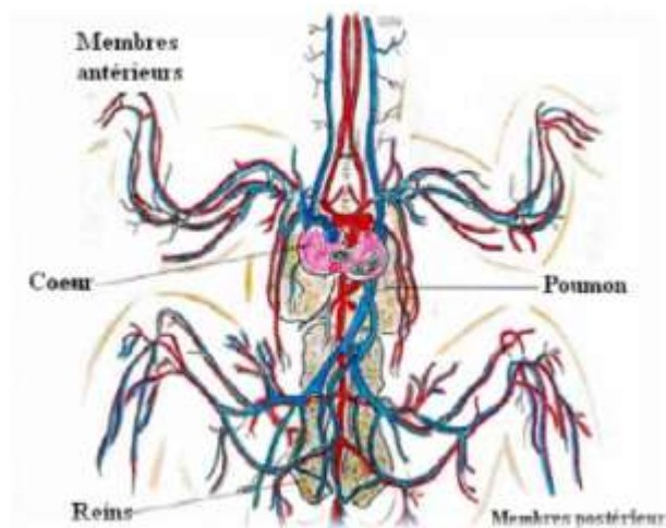
Figure 06: Appareil cardiovasculaire, système artérioveineux des oiseaux (Villate 2001)
