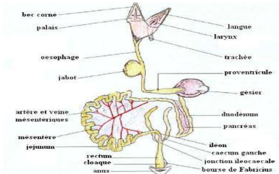
Figure 01: Vue latérale du tractus digestif du poulet (Villate, 2001)
