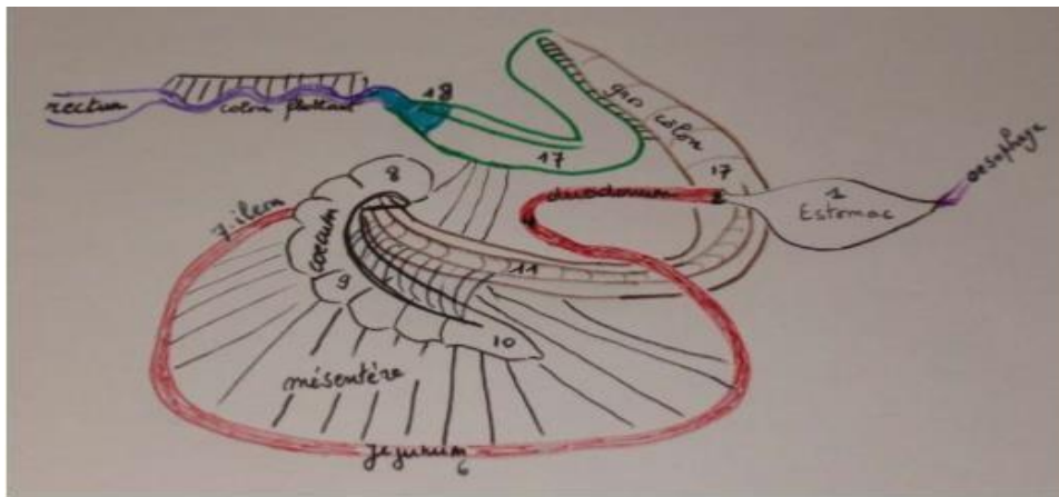
Figure (31) : SCHEMA DU TUBE DIGESTIF DU CHEVAL 1 estomac 2 3 4 5 duodénum 6 jéjunum 7 ileon 8 9 10 coecum 11 à 17 gros colon avec deux courbures (diaphragmatique et pelvienne) 18 colon transverse 19 20 colon flottant rectum.
