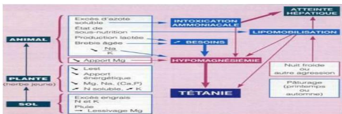
Figure2 : Physiopathologie de la tétanie hypomagnésémique. (Brugere ,2004)
