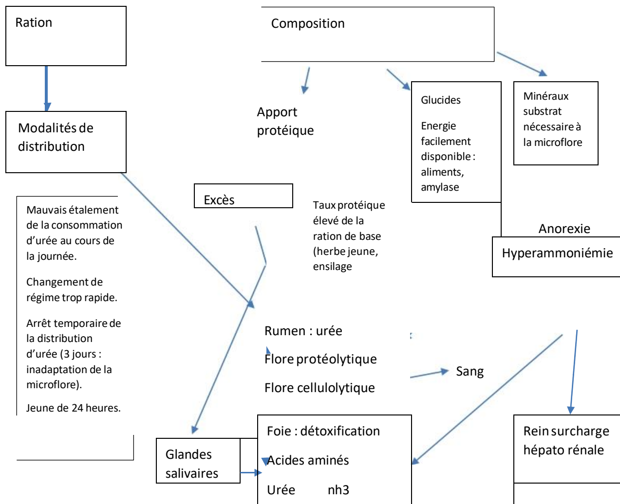
Figure4 : physio pathogénie de l'alcalose (Gourreau, Bendali ,2007)
